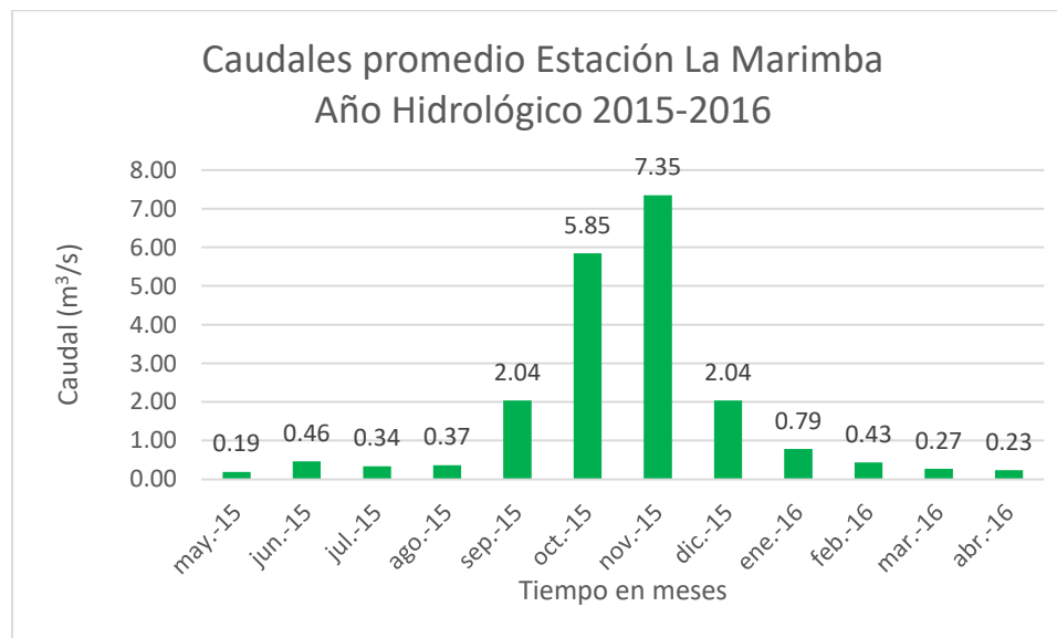
Figura 2. Caudales promedio de la Estación La Marimba para el año hidrológico 2015-2016.
