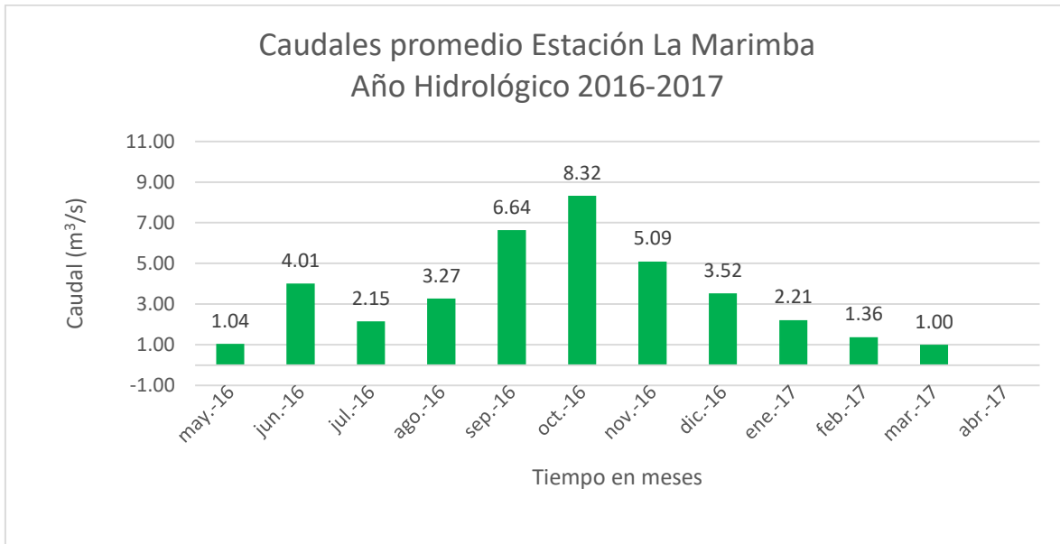
Figura 3. Caudales promedio de la Estación La Marimba para el año hidrológico 2016-2017.
