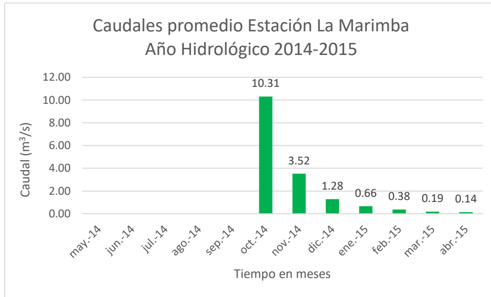
Figura 1. Caudales promedio de la Estación La Marimba para el año hidrológico 2014-2015. Los datos inician a partir del mes de octubre, momento en el que se instaló la Estación Hidro-Meteorológica
